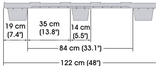
VISTA DEL LADO LARGO
