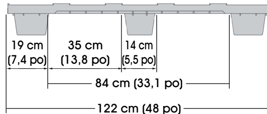
VUE DU CÔTÉ LONG
