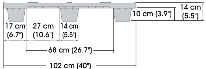
VISTA DEL LADO CORTO
