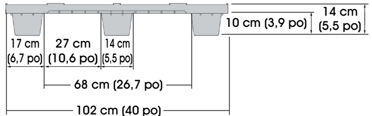
VUE DU CÔTÉ COURT
